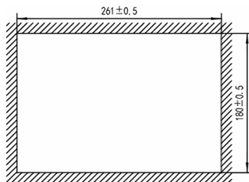
开孔尺寸
