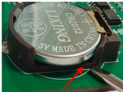
拆卸电池
