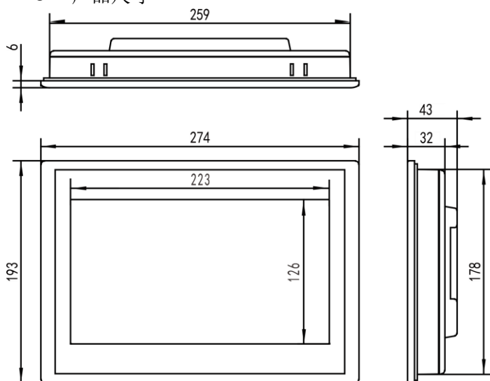
外形尺寸
