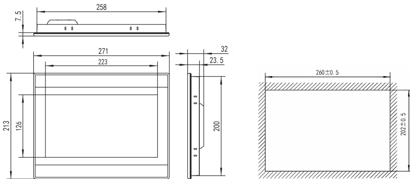
外形尺寸
