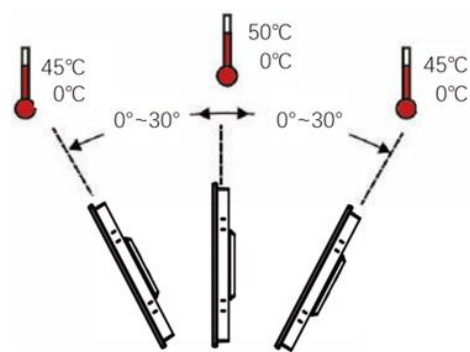
安装角度
