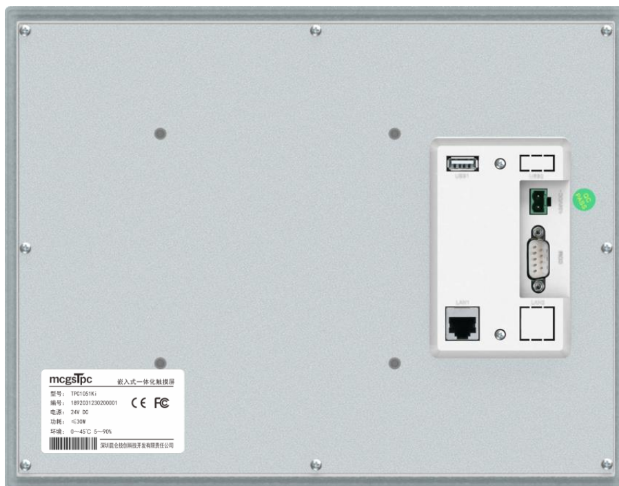
底视图
