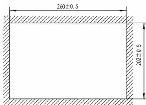
开孔尺寸
