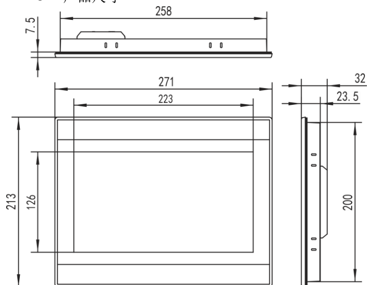
外形尺寸
