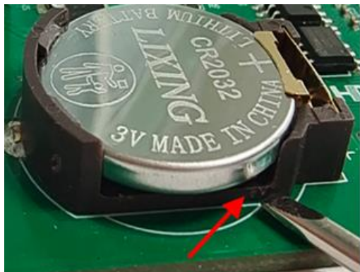
拆卸电池
