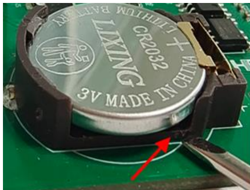
拆卸电池
