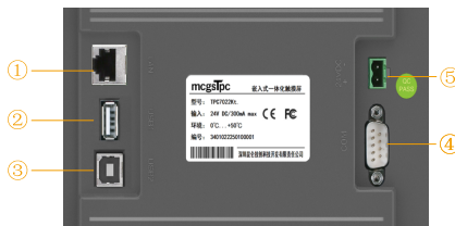
◎接口图
