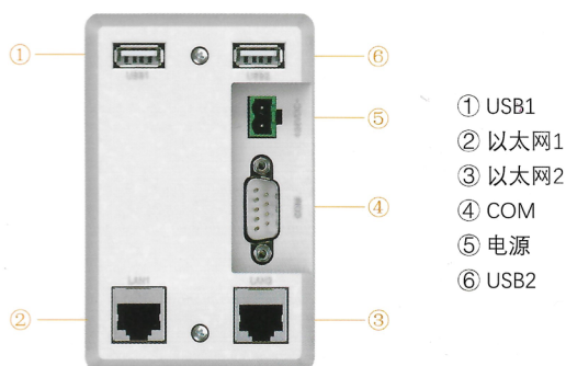
◎ 接口图
