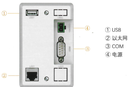
◎ 接口图
