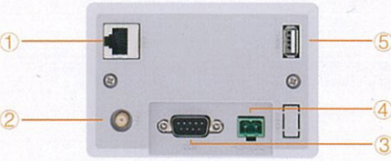
◎接口图
